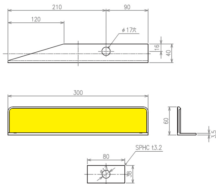
詳細図
