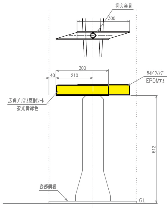
設置図
